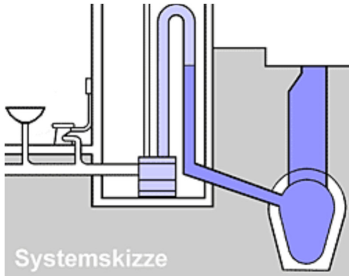
Hebeanlage
